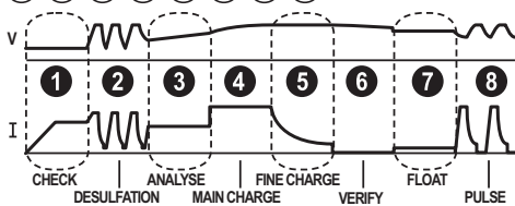
Fases de carga PULSE-TRONIC.
