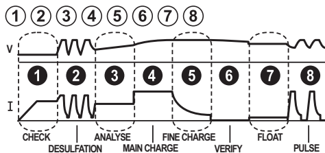
Фазы зарядки PULSE-TRONIC.
