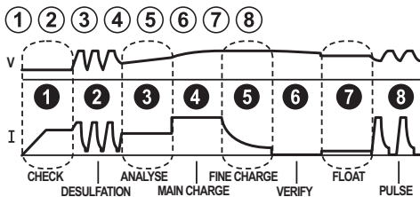
Фази на зареждане PULSE-TRONIC.
